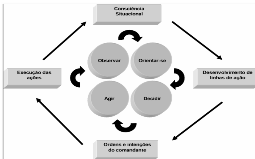
Figura 1 - Ciclo OODA
