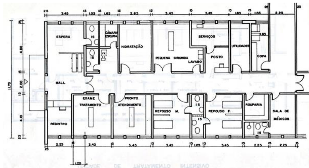
Imagem - Planta baixa do hospital. Fonte: Arquivo pessoal.
